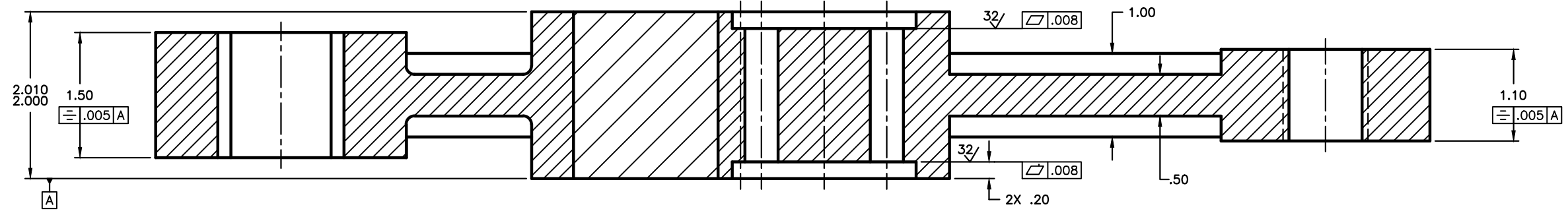
SECTION A-A
